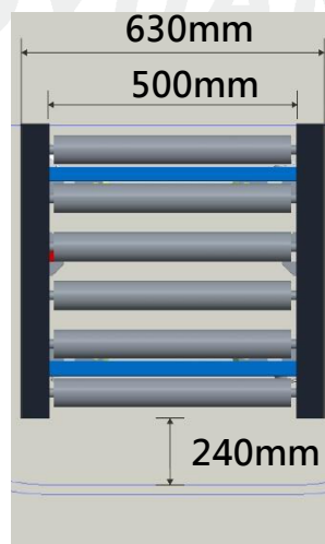
圖4滾台(單位:mm)
