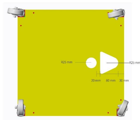
圖2貨架底板(單位:mm)
